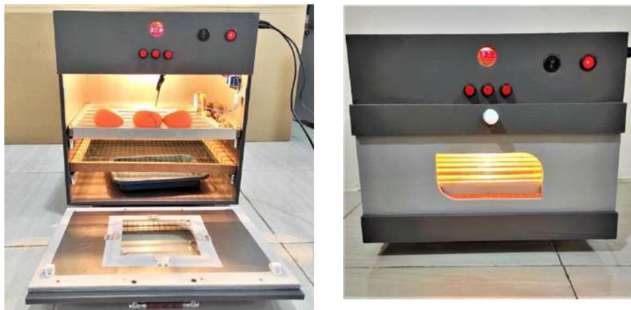
Gambar 5. Kandang Ayam Penetas Telur
